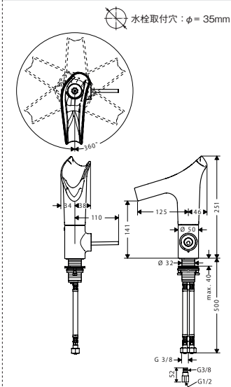
12112000 アクサースタルクV シングルレバー 混合水栓 140 (ポップアップ引棒無)
