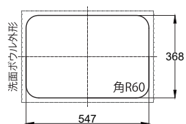
カウンター切欠図
