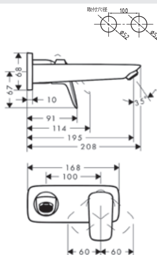
71220000 ロギス シングルレバー 洗面混合水栓 壁付式195(化粧部)
