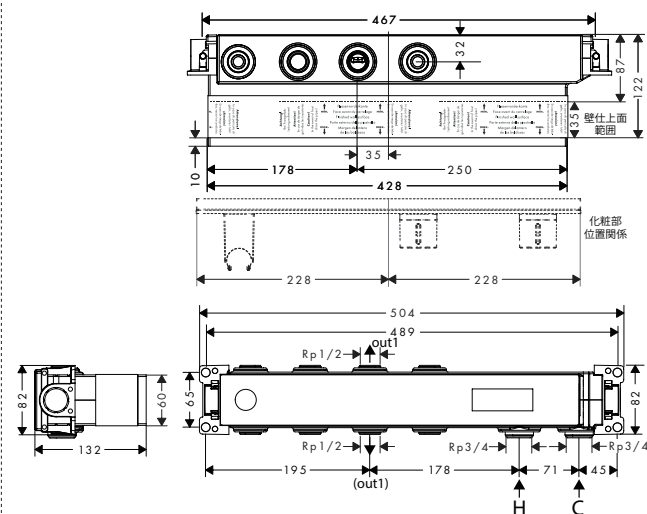
18312180 サーモスタットモジュールセレクト 4アウトレット用(埋込部)
