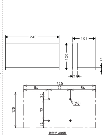
40873000 アクサー シャワーコレクション ロングシェルフ 24/12
