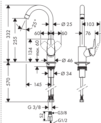
72810000 タリス S シングルレバーキッチン混合水栓 ハイスパウト 260
