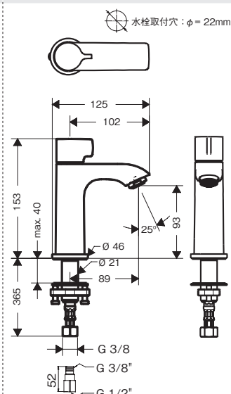
71120000 ロギス 単水栓 70 (ポップアップ引棒無) [一般地・寒冷地共用形]
