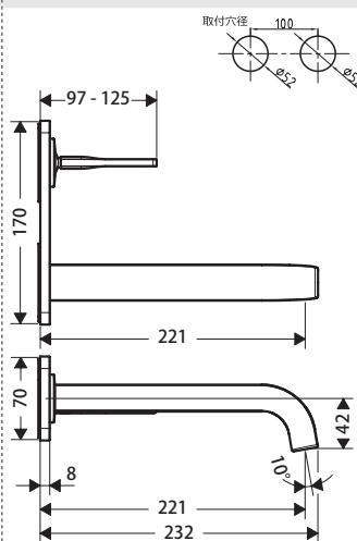
36114000 アクサー・チッテリオE シングルレバー 壁付式洗面混合水栓 220(プレート付)
